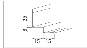
Nr. 50/15 0,5 mm dick
