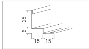
Nr. 50/14 0,5 mm dick
