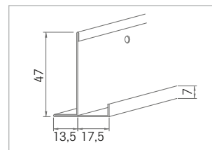
Nr. 8030/15 15er Platte 0,6 mm dick
