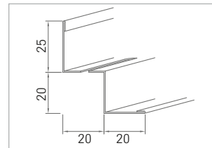
Nr. 56/35 0,6 mm dick (mit Lüftungsschlitzen)
