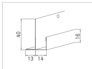
Nr. 8030/13 13er Platte 0,5 mm dick
