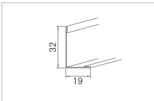
Nr. 51/32G 0,5 mm dick
