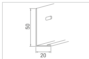
Nr. 51/20 1,0 mm dick
