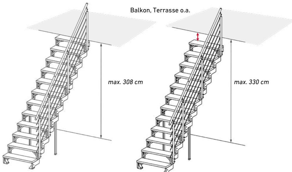
Abbildung 1: 2-14 Stufen
