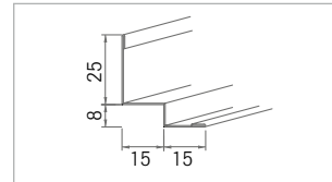
Nr. 50/15G 0,5 mm dick
