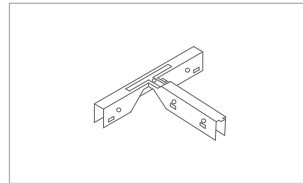
Nr. 61/2 T-Verbinder
