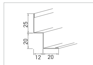
Nr. 56 0,6 mm dick
