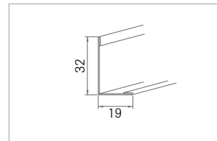
Nr. 51/32G 0,5 mm dick
