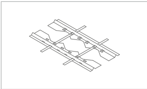
Nr. 8069/1*, 8069/0*, 8069/3, 8069/2, 8069/4 Montagerahmen
