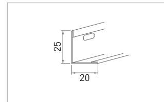
Nr. 53 0,6 mm dick
