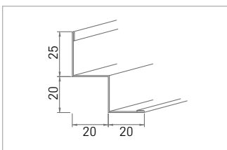
Nr. 56/20 0,6 mm dick Nr. 56/21 1,0 mm dick Nr. 56/23 1,5 mm dick
