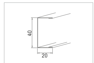
Nr. 57 0,5 mm dick
