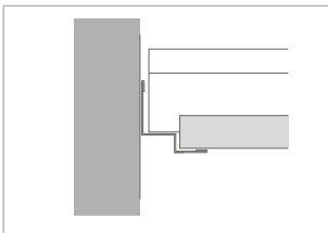
Nr. 50/14, Nr. 50/15G Contura-Decken
