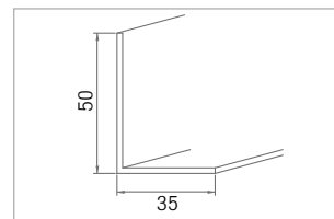
Nr. 51/02 2,0 mm dick
