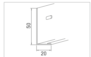
Nr. 51/20 1,0 mm dick
