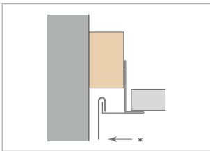
Nr. 8030/15
