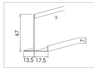
Nr. 8030/15 15er Platte 0,6 mm dick
